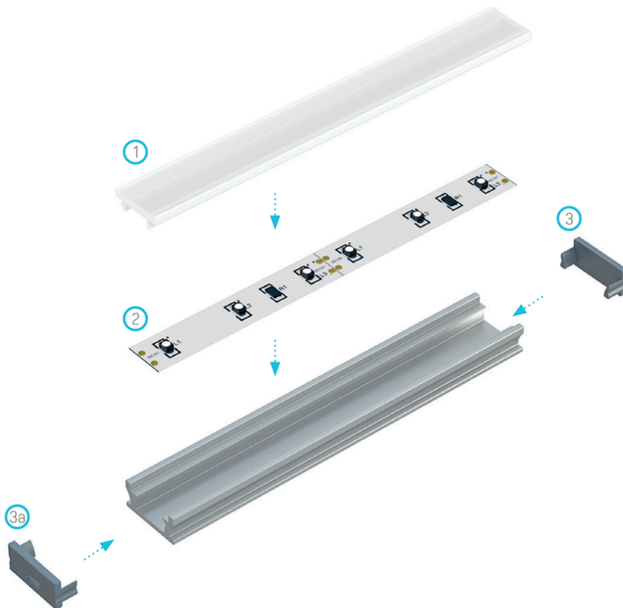
Schema di montaggio degli elementi del sistema di illuminazione con l'uso del profilo "Zeno" e (1) del diffusore calpestabile, (2) di due strisce LED, (3) del tappo senza foro, (3a) del tappo con foro.
